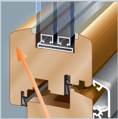
Nahtloser Übergang vom Fensterflügel zur Scheibe, keine Glasleiste mehr erforderlich
