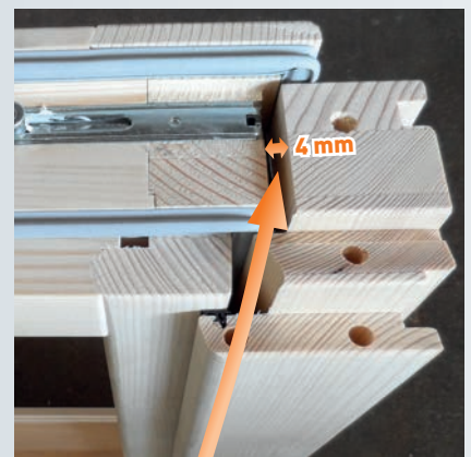
Nur 4 mm Falzluft! Möglich durch das eingefräste Schließblech: Perfekt als Einbruchschutz
